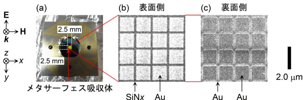
図 2 厚さ 100 nm の窒化シリコン(SiNx)膜を用いて作製した赤外線吸収メタサーフェス
